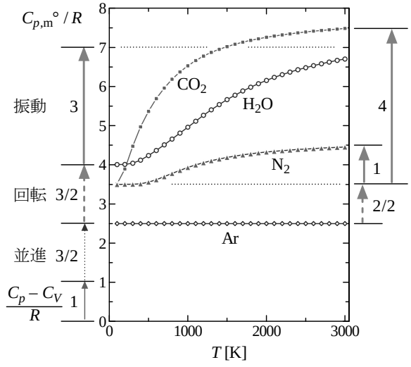
図 3.4: 定圧モル熱容量への分子運動の寄与
