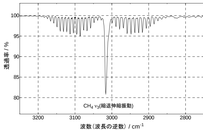
メタン ν₃ 帯の吸収スペクトル
