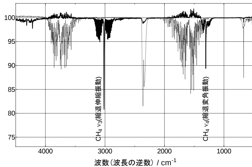
メタン・大気赤外吸収スペクトル
