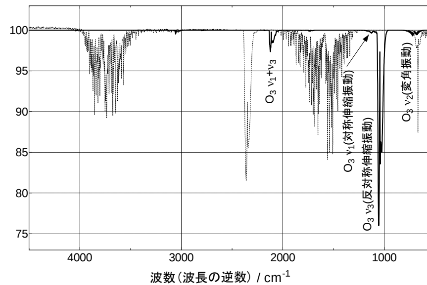
オゾン・大気赤外吸収スペクトル
