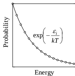
図 6.1 ボルツマン分布
