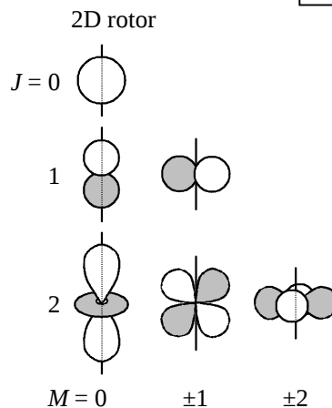
図 6.2 回転波動関数と多重度
