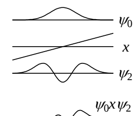
図 2.5b 禁制遷移
