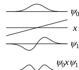
図 2.5a 許容遷移
