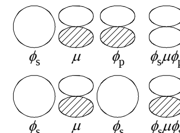
図 5.4 \Delta l 選択則
