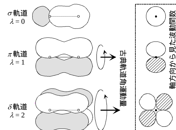
図 5.5 分子軌道
