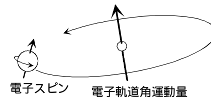
図 5.2 スピンと軌道角運動量
