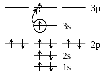
図 5.1 Na-D 線の電子遷移
