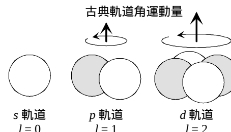
図 5.3 原子軌道
