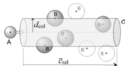
図 1.2 衝突断面積と衝突頻度
